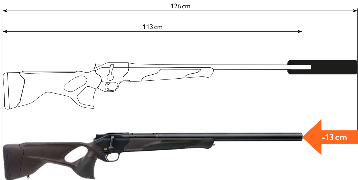
R8 Ultimate im Kaliber .300 Win. Mag. , Lauflänge 65 cm, Over-Barrel Schalldämpfer vs. R8 Ultimate Silence im Kaliber 8,5x55 Blaser , Lauflänge 47 cm, Integralschalldämpfer
